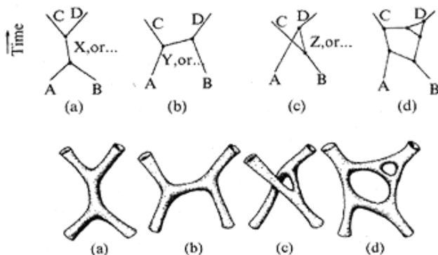
شکل 14 - دیگرهای فین من در تئوری ذرات نقطه‌ای (بالا) و تئوری رشته‌ها (پائین).
