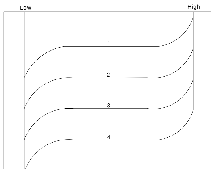
شکل ۱۱ مشخصه دما - زمان یک سیستم ترموکلین [۷]
